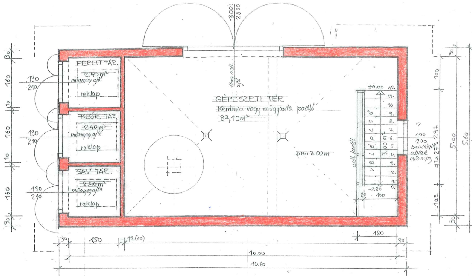
FÖLDSZINTI ALAPRAJZ 1=50
