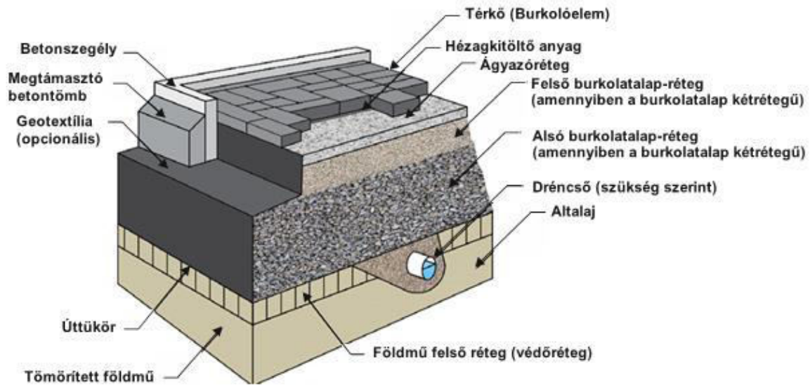
1. ábra – Kiselemes burkolatú útszerkezet (továbbiakban: terkő szerkezet)
