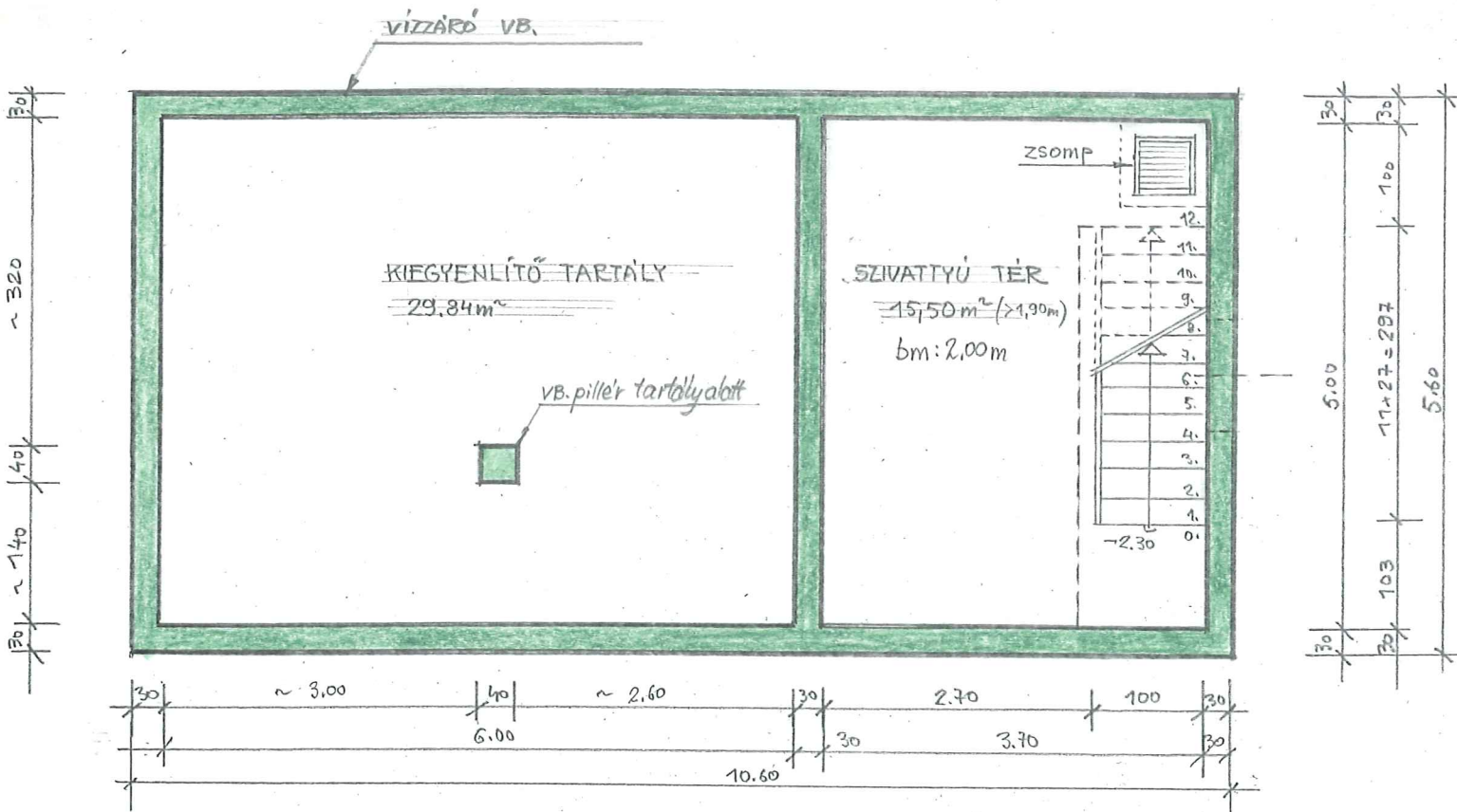
PINCE ALAPRAJZ 1=50
