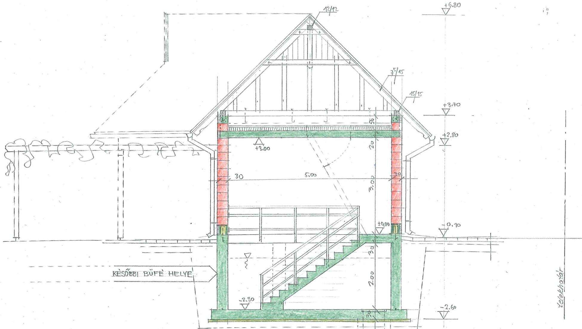
KERESZTMETSZET 1:50
