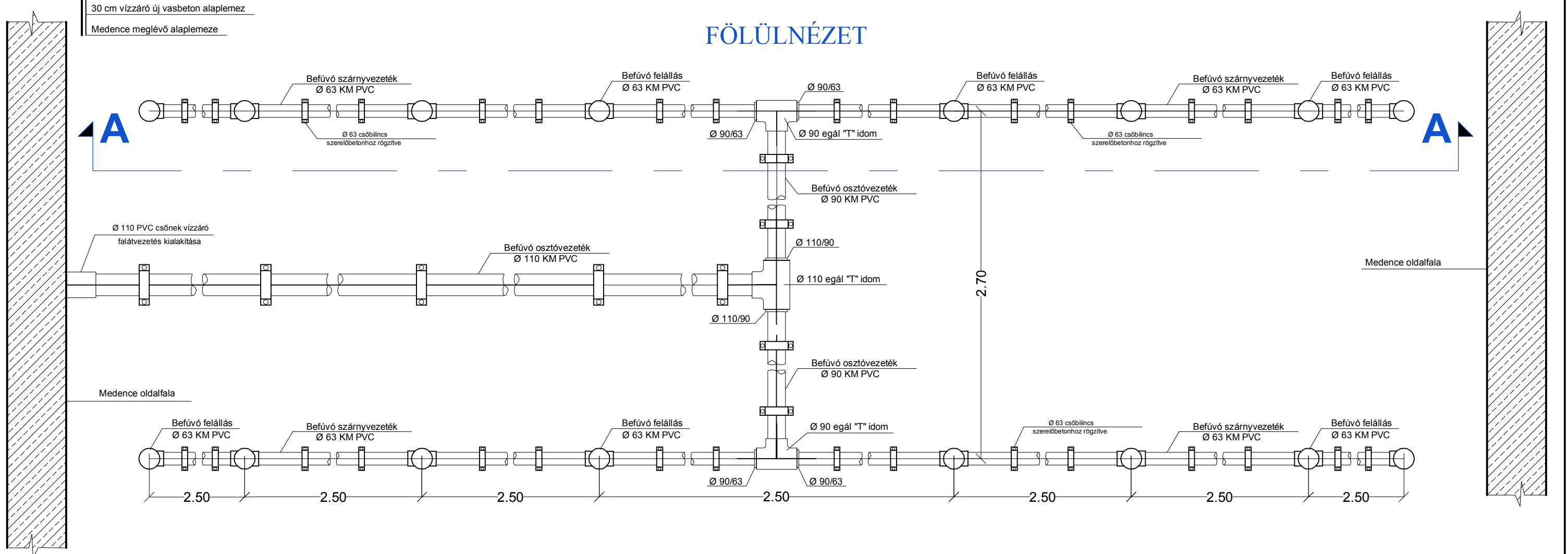
Befúvók végleges kialakítása
