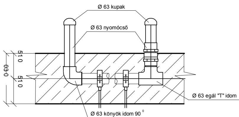
Befúvó felállás kialakítása betonozáskor
