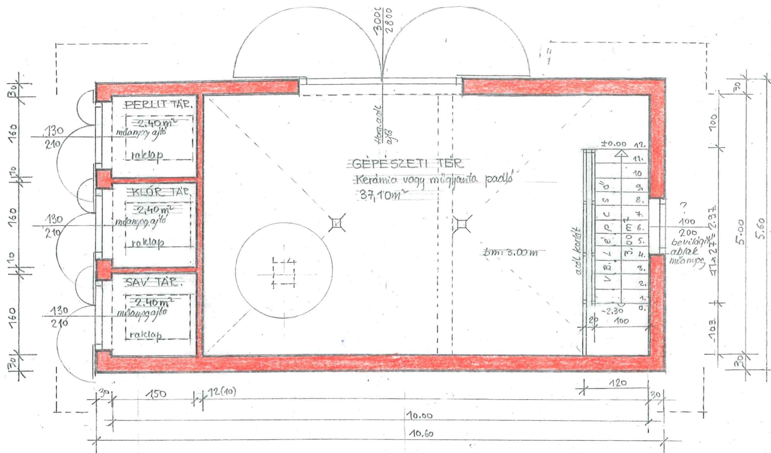
FÖLDSZINTI ALAPRAJZ 1=50
