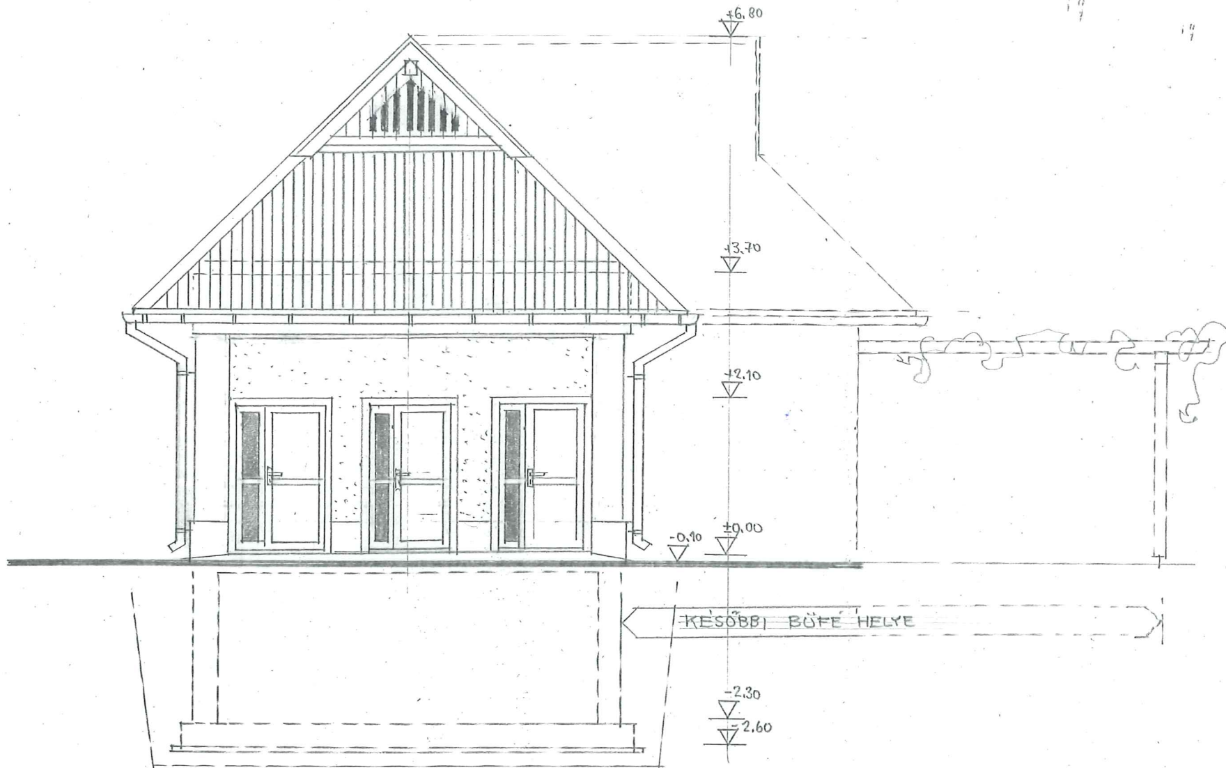
OLDALSÓ HOMLOKZAT 1:50
